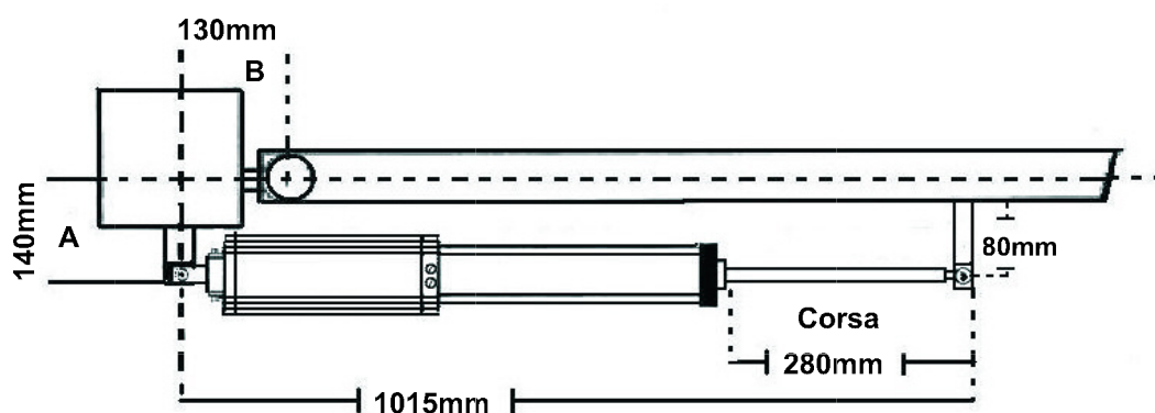
Fig.4 Corsa Stelo 280mm con rallentamento
