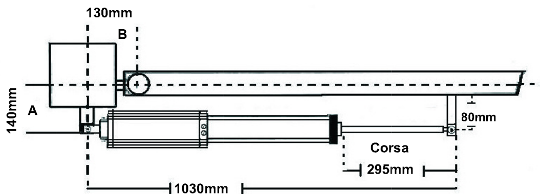
Fig.5 Corsa Stelo 295mm senza rallentamento
